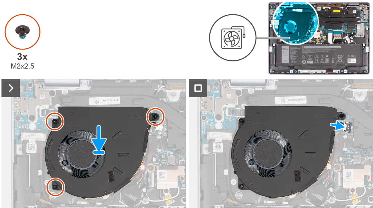
Figure 26. Installing the fan
