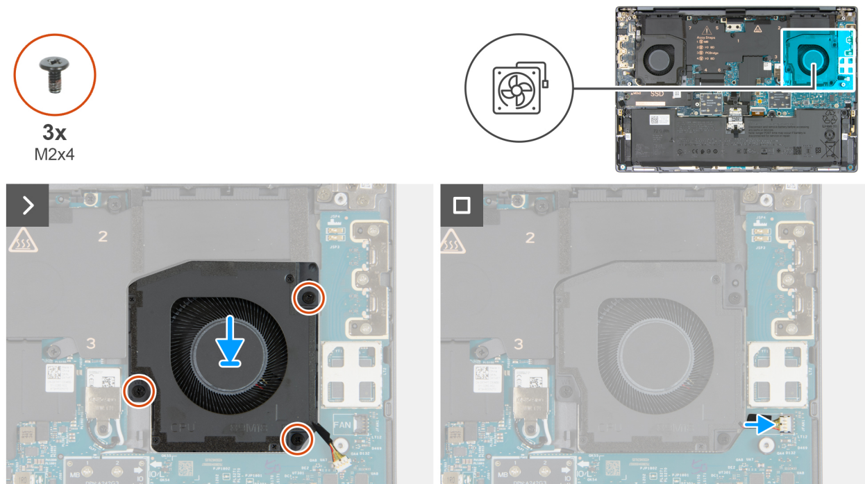
Figure 28. Installing the left fan
